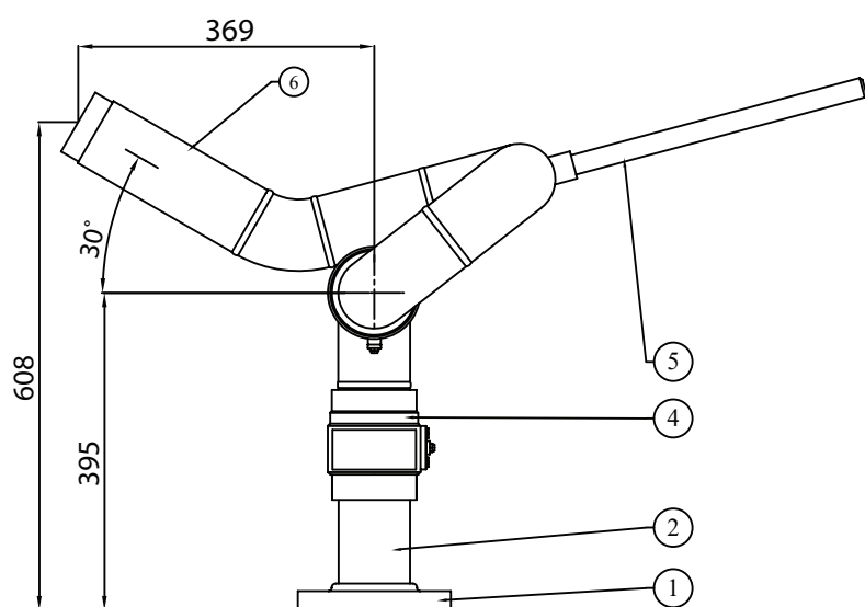
ELEVATION
